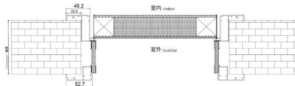
同色铝框 - 平面结构图 Plan structure diagram
